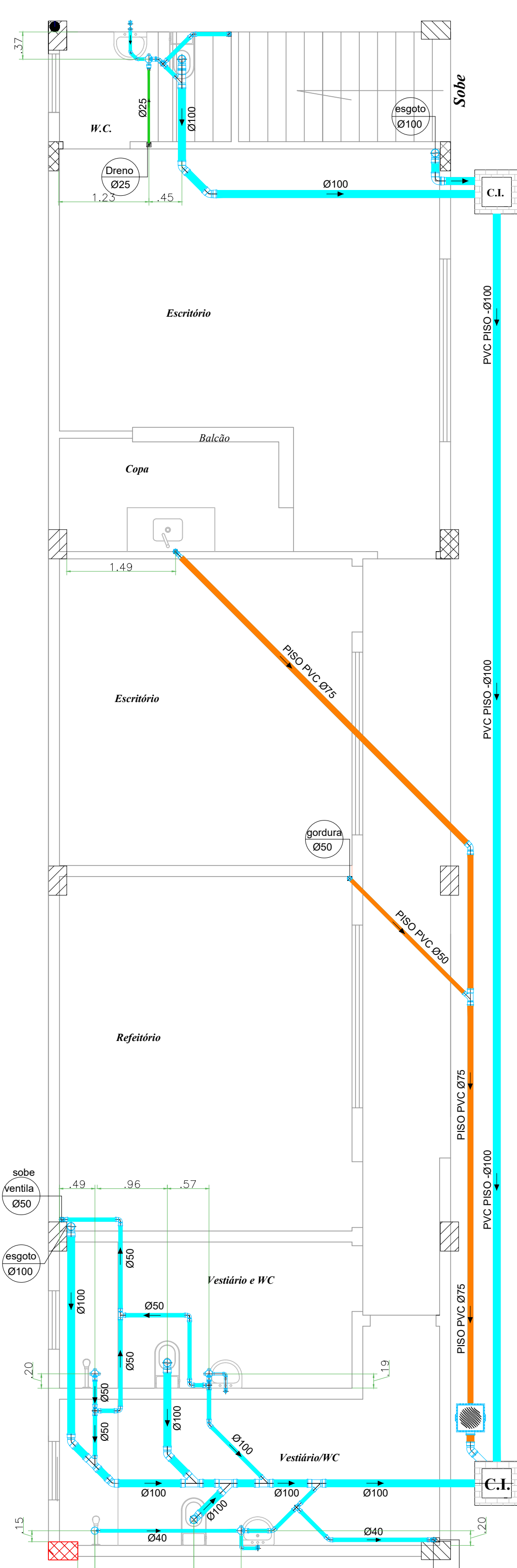
PLANTA - BAIXA GALPÃO - 03
