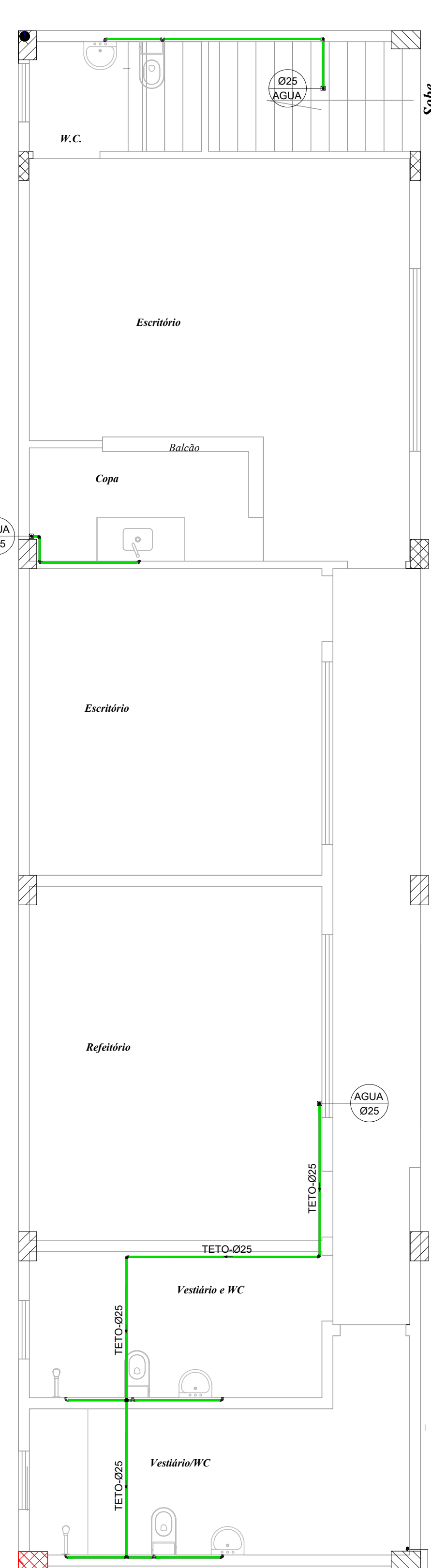
PLANTA - BAIXA GALPÃO - 03-AGUA FRIA
